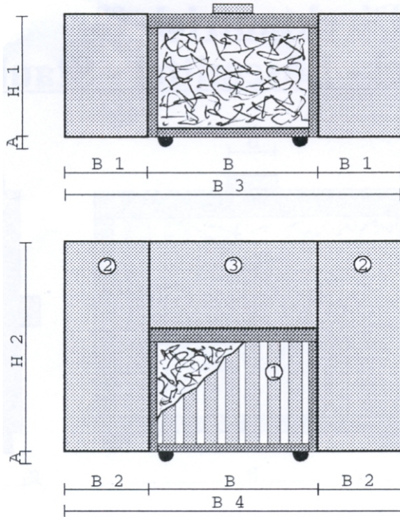
Abbildung zeigt ein Gerät (Typ RD) mit Filtermatte und arretierbaren Seitenblechen
